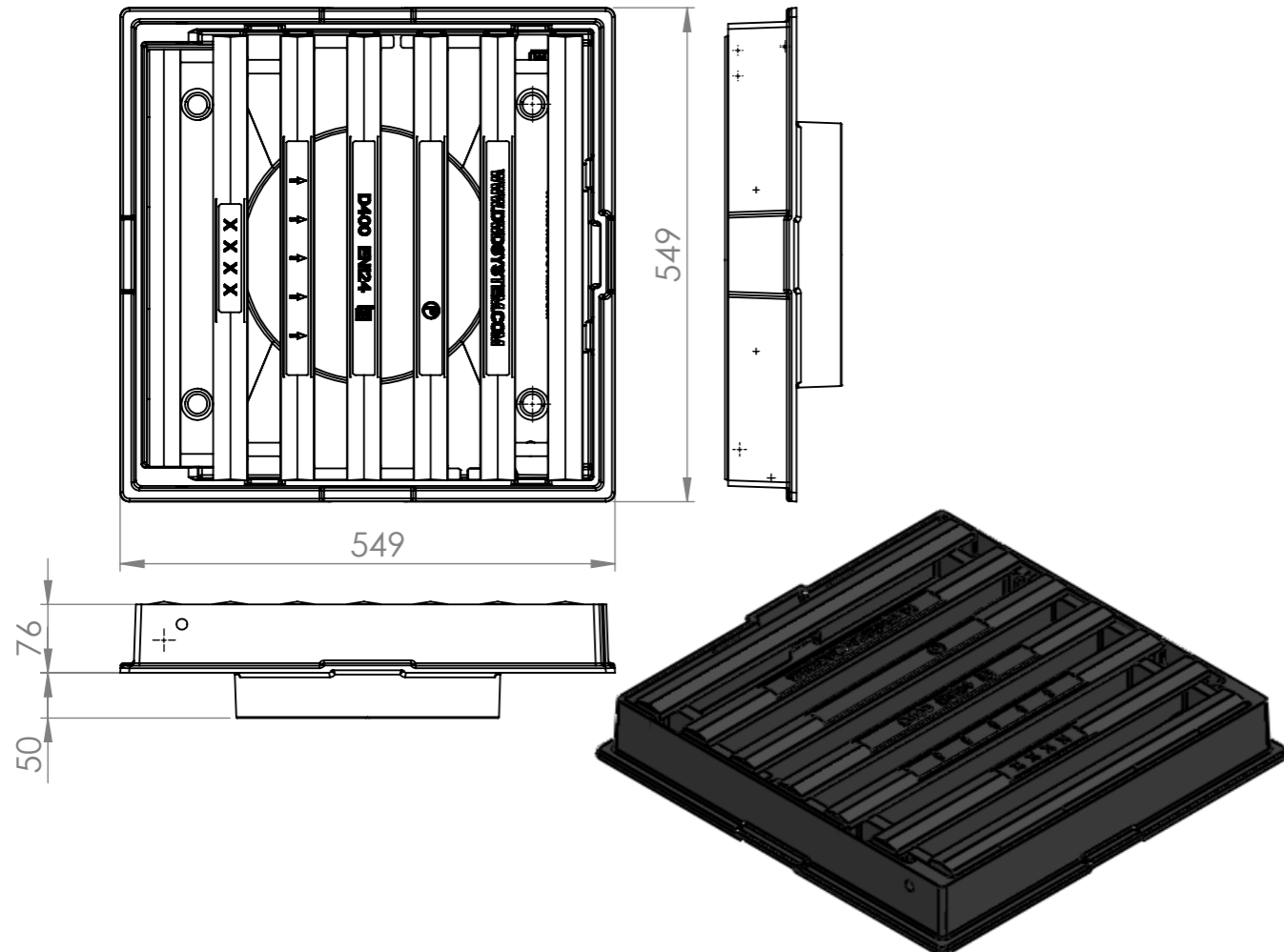
Zwieńczenie 500x500 WM-Z-500x500
