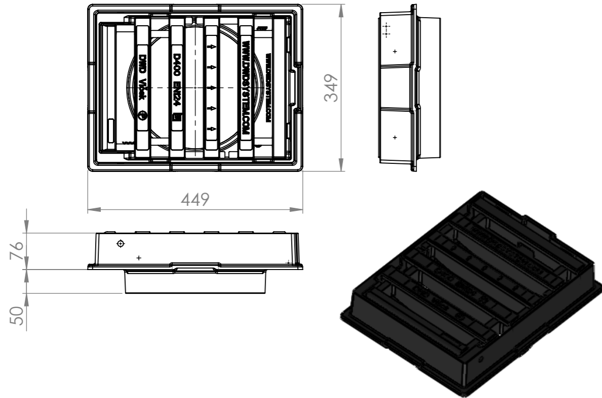
Zwieńczenie 300x400 WM-Z-300x400
