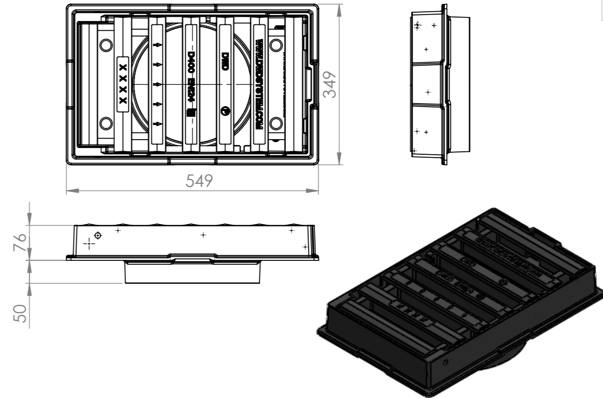
Zwieńczenie 300x500 WM-Z-300x500
